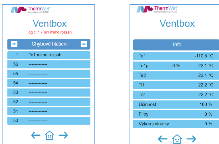
Obrázek 30: Příklad poruchy – Chyba čidla_Te1
