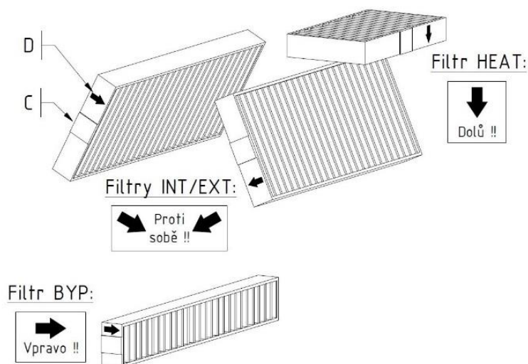
Obrázek 27: Vytahovací páska a směr montáže filtru (LEVÁ varianta)
