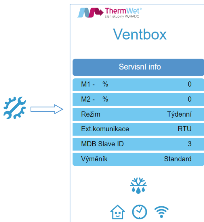
Obrázek 10: Servisní informace
