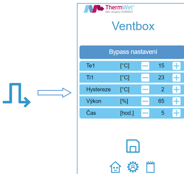
Obrázek 19: Bypass nastavení
