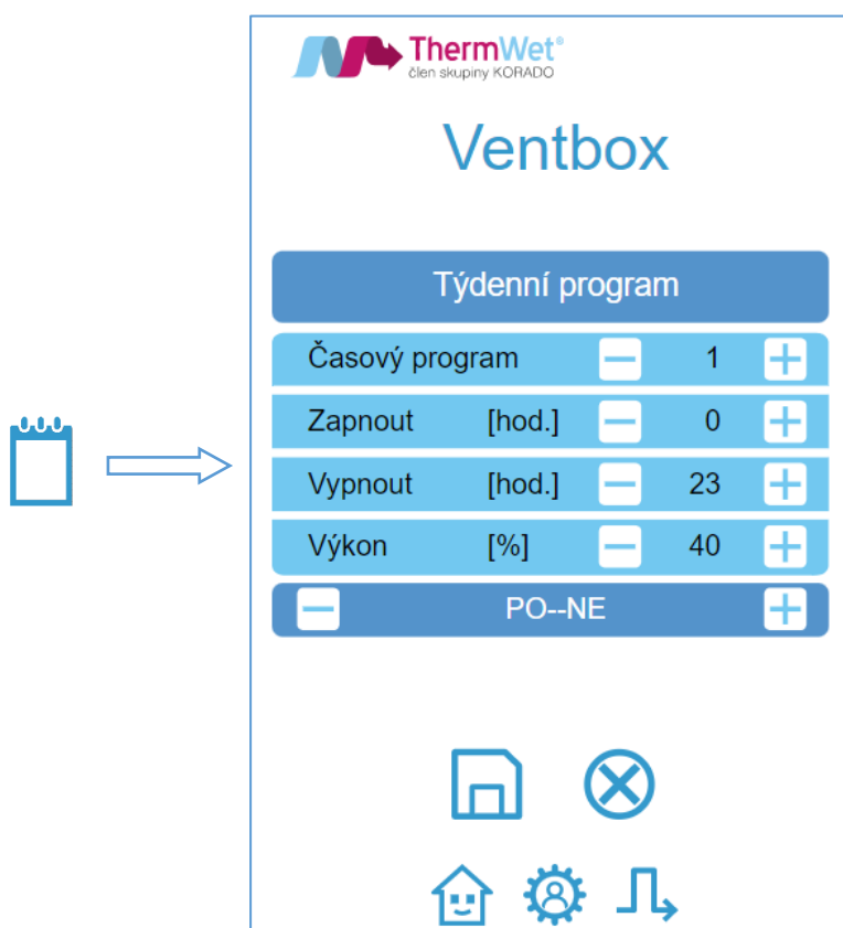
Obrázek 18: Týdenní program
