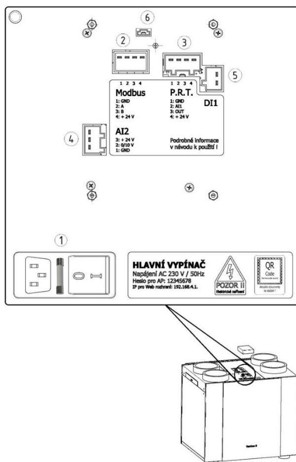
Obrázek 33: Panel řízení s připojením pro konektory
