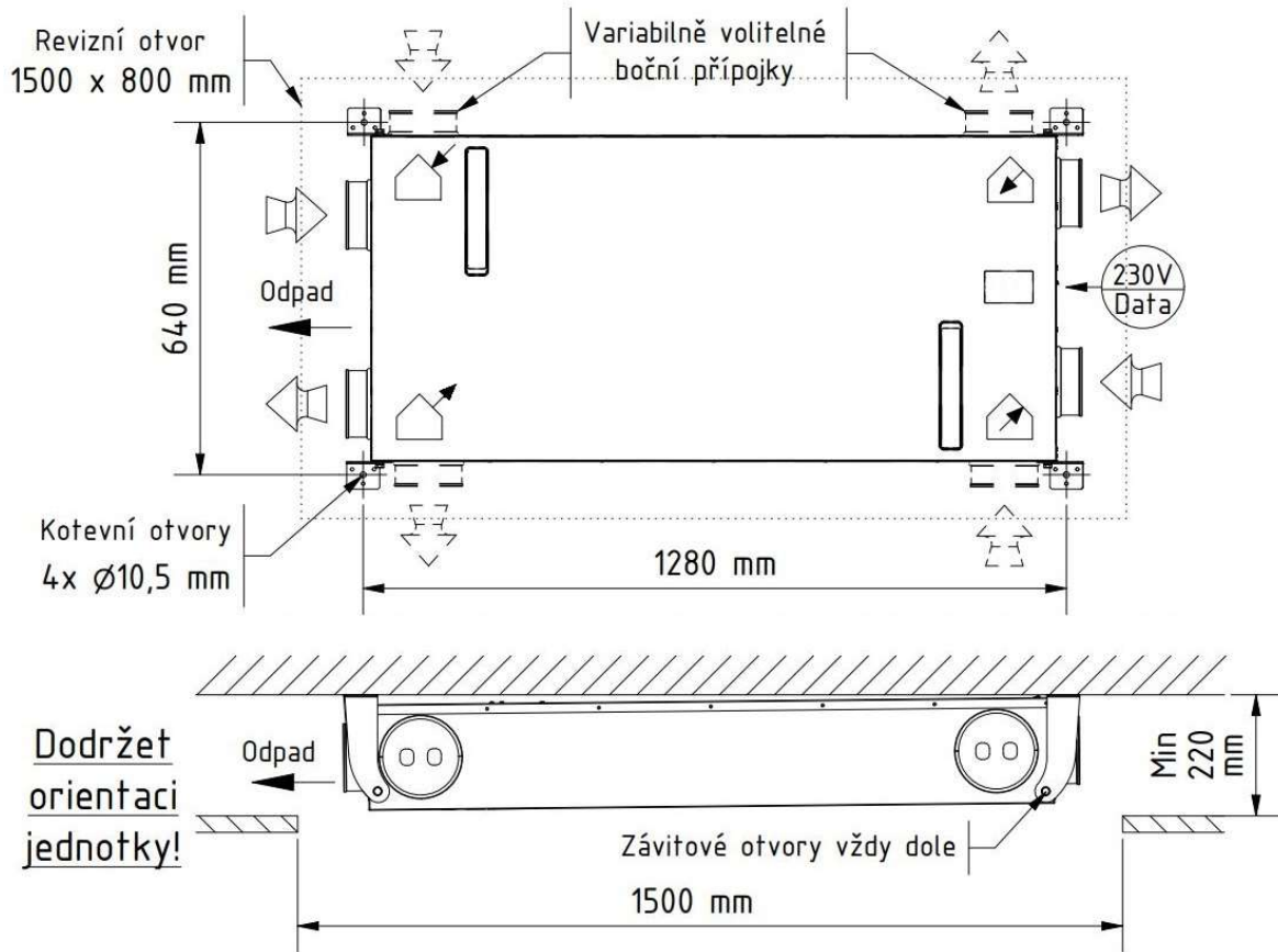
Obrázek 32: Instalační prostor pro „Podstropní montáž“
