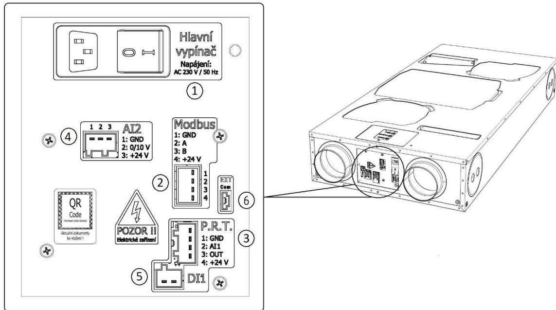
Obrázek 34: Panel řízení s připojením pro konektory
