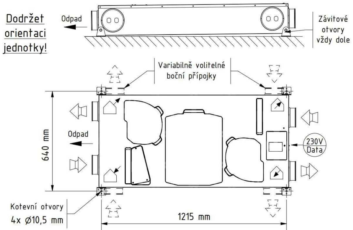
Obrázek 31: Instalační prostor pro „Podlahovou montáž“
