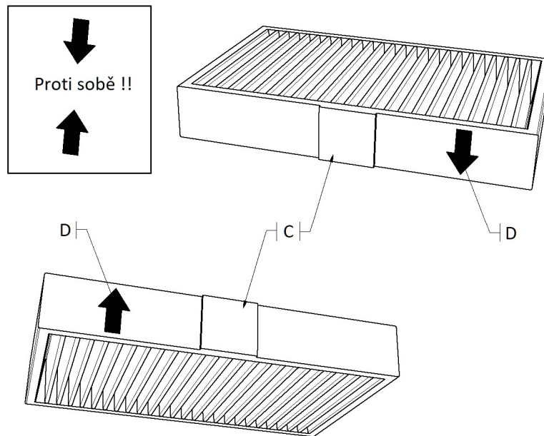
Obrázek 27: Vytahovací páska a směr montáže filtru
