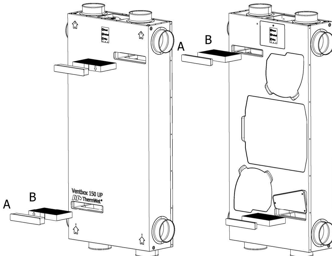
Obrázek 26: Vyjmutí filtru (LEVÁ / PRAVÁ varianta)
