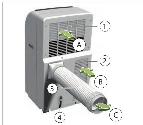
Obr. 2: Pohled zezadu
