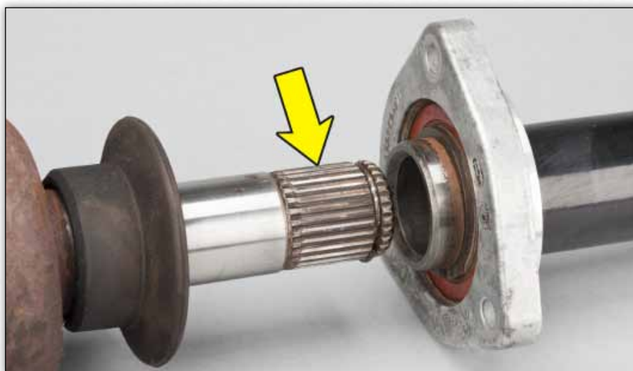
Obrázek 1: Místo nanesení maziva na spoj hnací hřídele
